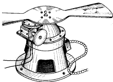
Рис. 12. Обтюратор со счетчиком числа оборотов
