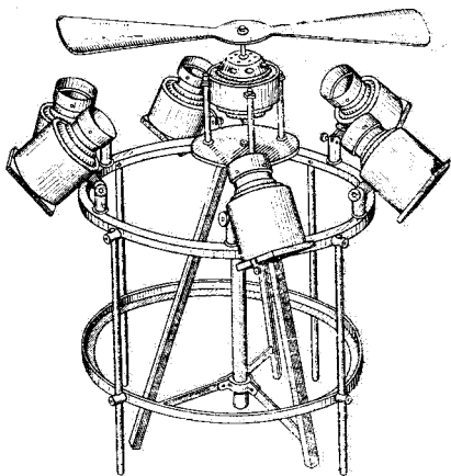
Рис. 11. Устройство фотографического метеорного патруля. Симферопольская метеорная станция
