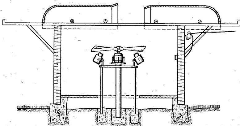
Рис. 13. Схема устройства павильона для метеорного патруля
