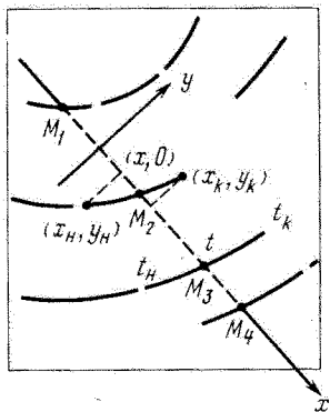
Рис. 15. Измерение фотографии метеора и определение координат опорных точек
