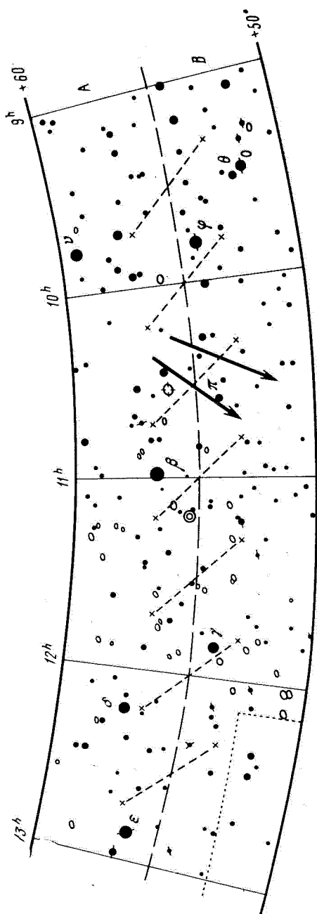
Рис. 8. Полоса карты для наблюдений высот телетеоретов, Атлас А. Бечвара. Область Большой Медведицы
