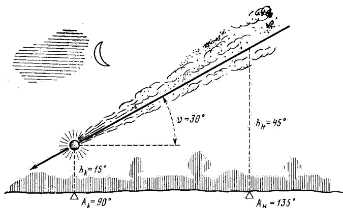
Рис. 17. Элементы видимой траектории болида
