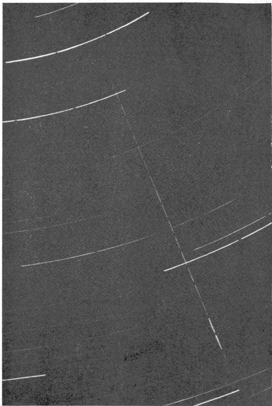
Рис. 14. Базисный фотоснимок метеора. Крымская станция ВАГО
