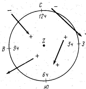
Рис. 7. Определение положения ( \pm ) и направления метеоров по «правилу циферблата»
