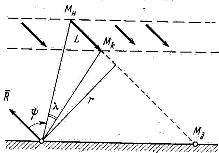
Рис. 2. Элементы траектории метеорного тела в атмосфере Штрихами ограничен метеорный слой в атмосфере
