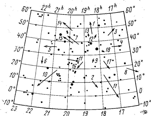
Рис. 3. Нанесение метеоров на карту атласа А. А. Михайлова
