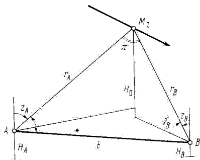
Рис. 16. Определение высоты некоторой точки на траектории метеора
