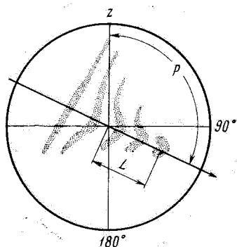
Рис. 9. Дрейф следа метеора относительно поля зрения трубы
