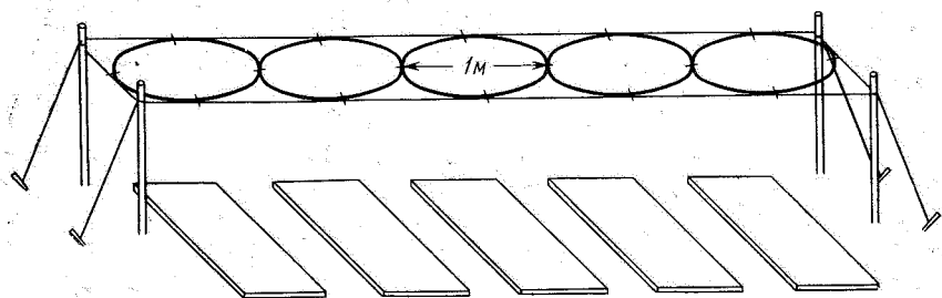
Рис. 6. Рамка для счета метеоров для пяти наблюдателей, располагающихся рядом
