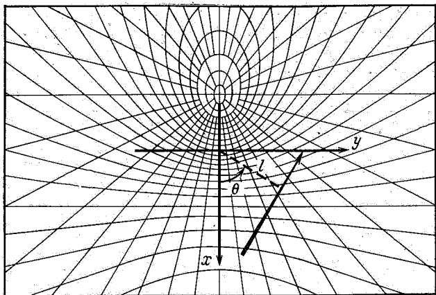
Рис. 4. Сетка Лоренцони. Параллели нанесены через 5^\circ , меридианы через 10^\circ
