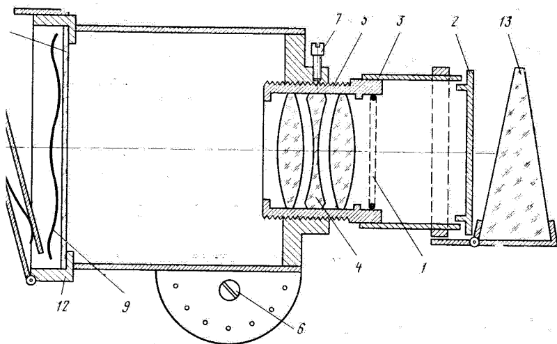
Схема устройства камеры для фотографирования метеоров
